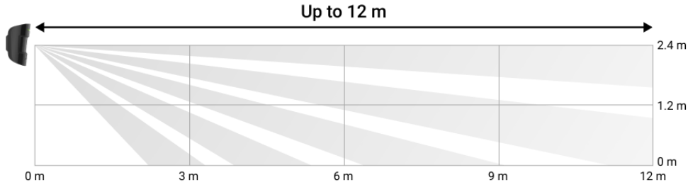
Dedektörün dikey görüş açısı
