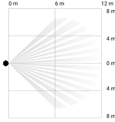
Dedektörün yatay görüş açısı
